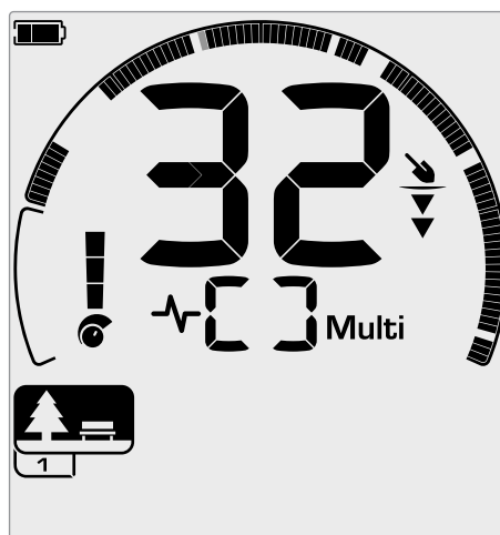
Пример, показывающий обнаружение принятой цели из цветных металлов с идентификатором цели 32. Сегмент 32 на шкале распознавания будет мигать.
